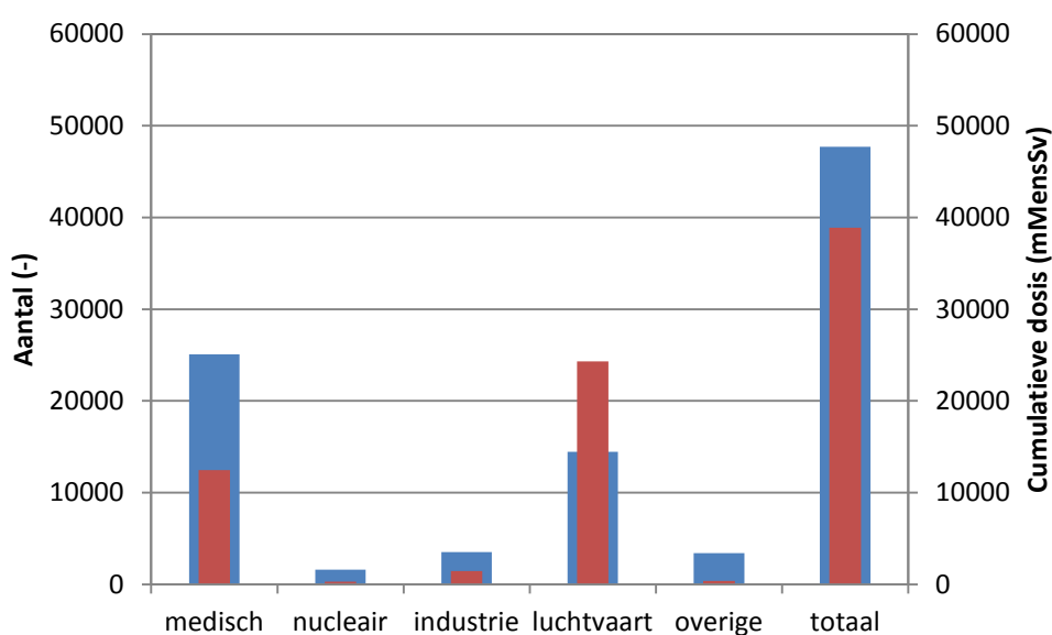
Figuur 1 Totaal aantal actieve geregistreerde personen ■ en bijbehorende cumulatieve dosis ■ met onderverdeling naar sector (2015).
