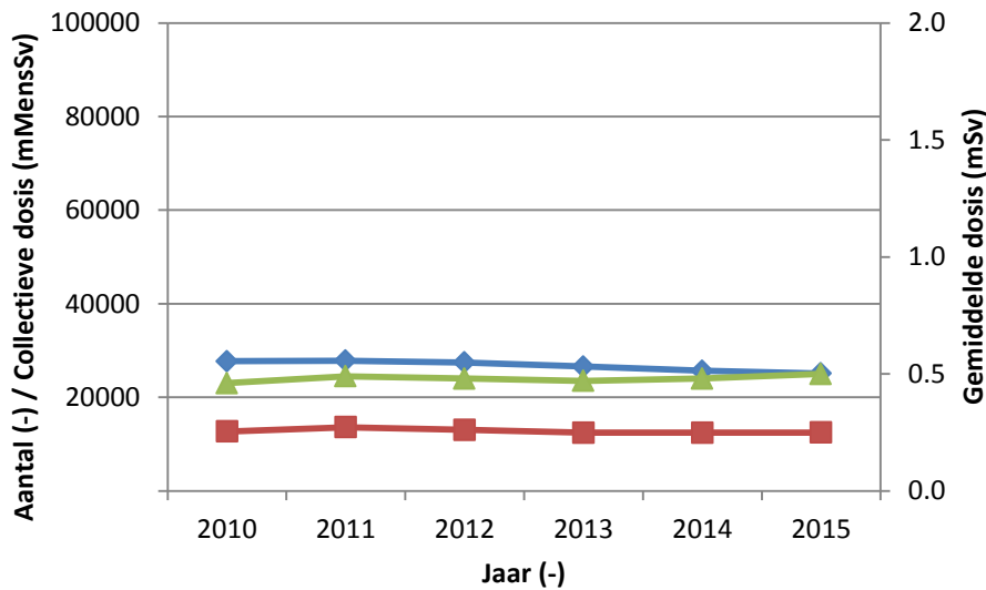
Figuur 3 Totaal aantal personen ( N ) ♦, de collectieve dosis ( S ) ■ en de gemiddelde dosis ( E_{Avg} ) ▲ voor de periode 2010 tot 2015 voor de medische sector.
