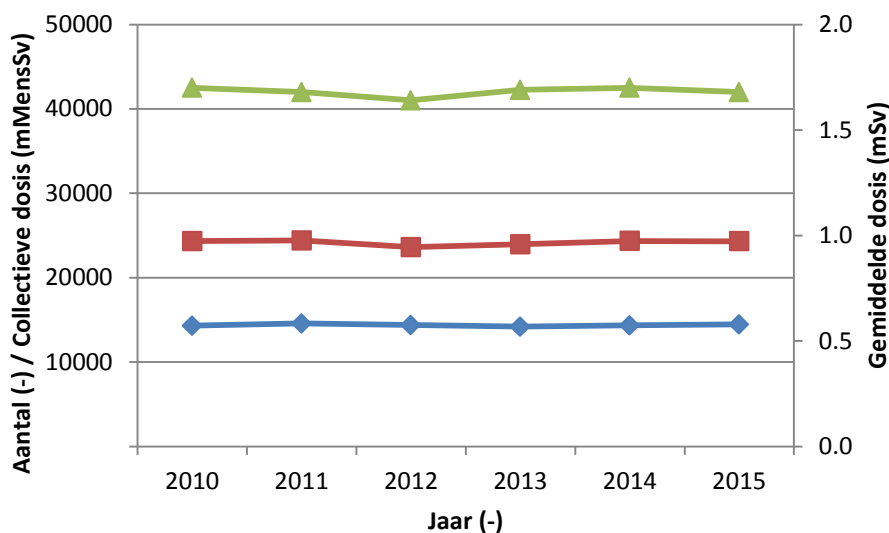
Figuur 6 Totaal aantal personen ( N ) ♦, de collectieve dosis ( S ) ■ en de gemiddelde dosis ( E_{Avg} ) ▲ voor de periode 2010 tot 2015 voor de luchtvaart sector.
