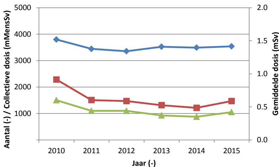
Figuur 5 Totaal aantal personen ( N ) ♦, de collectieve dosis ( S ) ■ en de gemiddelde dosis ( E_{Avg} ) ▲ voor de periode 2010 tot 2015 voor de industriële sector.
