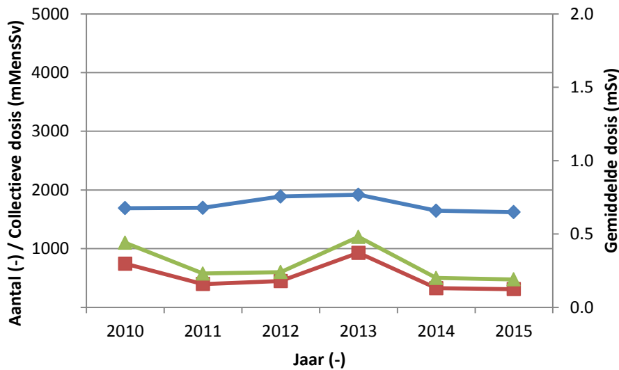
Figuur 4 Totaal aantal personen ( N ) ◆, de collectieve dosis ( S ) ■ en de gemiddelde dosis ( E_{Avg} ) ▲ voor de periode 2010 tot 2015 voor de nucleaire sector.
