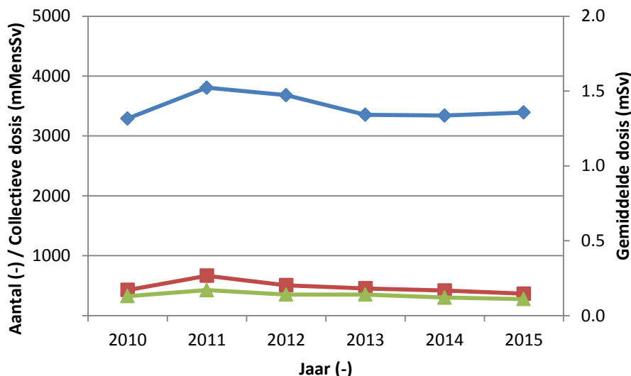
Figuur 7 Totaal aantal personen ( N ) \blacklozen , de collectieve dosis ( S ) \blacksquare en de gemiddelde dosis ( E_{Avg} ) \blacktriangle voor de periode 2010 tot 2015 voor de overige sectoren.
