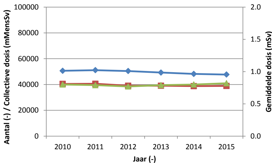
Figuur 2 Totaal aantal personen ( N ) ♦, de collectieve dosis ( S ) ■ en de gemiddelde dosis ( E_{Avg} ) ▲ voor de periode 2010 tot 2015 voor alle sectoren tezamen.
